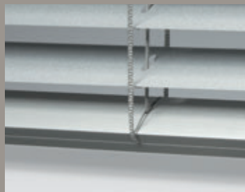
Ladderkoord of ladderband worden in de onderlat weggewerkt.
