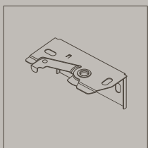
Universele schaarsteun Scala 25 (alu 16, 25 en 35 mm) 2208 0100 verzinkt 2208 0101 wit 2208 0102 beige 2208 0103 antraciet
