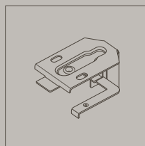
Universele schaarsteun Scala 50 (alu 50 en 70 mm) 2308 0000 verzinkt 2308 0001 wit 2308 0002 beige 2308 0003 antraciet
