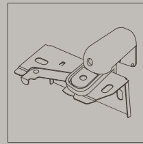
Klemsteun kunststofraam boven (wit) Scala 25 (16 & 25 mm) 2208 0300 verzinkt 2208 0301 wit 2208 0302 beige 2208 0303 antraciet
