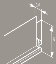
onderlijst kleine cassette
