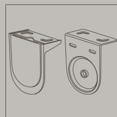
Montagesteun Type 7070/7080 niet commando zijde (standaard)
