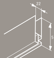
onderlijst grote cassette
