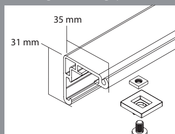
Afmetingen montageprofiel
